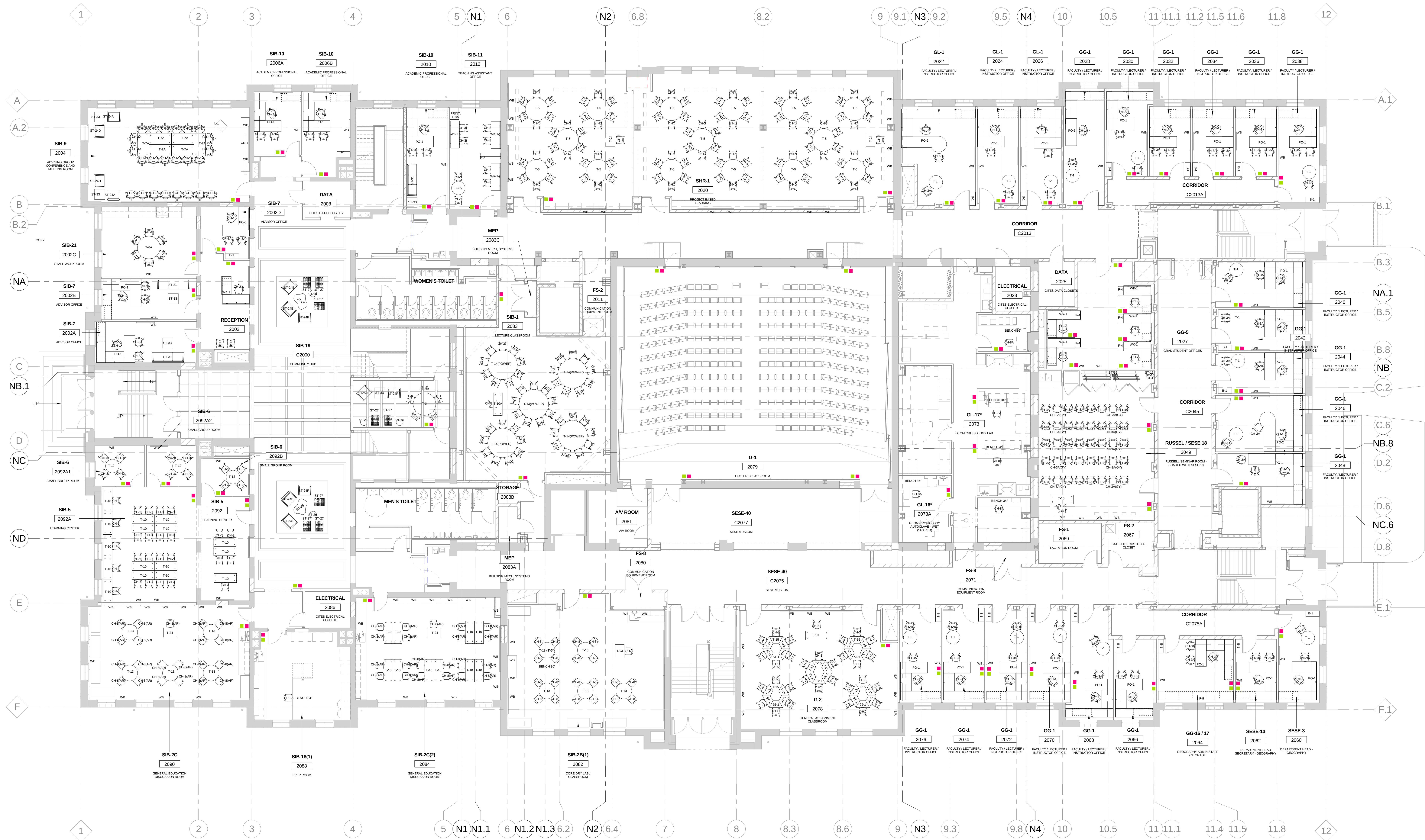
1 LEVEL 2 - FURNITURE SCALE: 1/8" = 1'-0"
