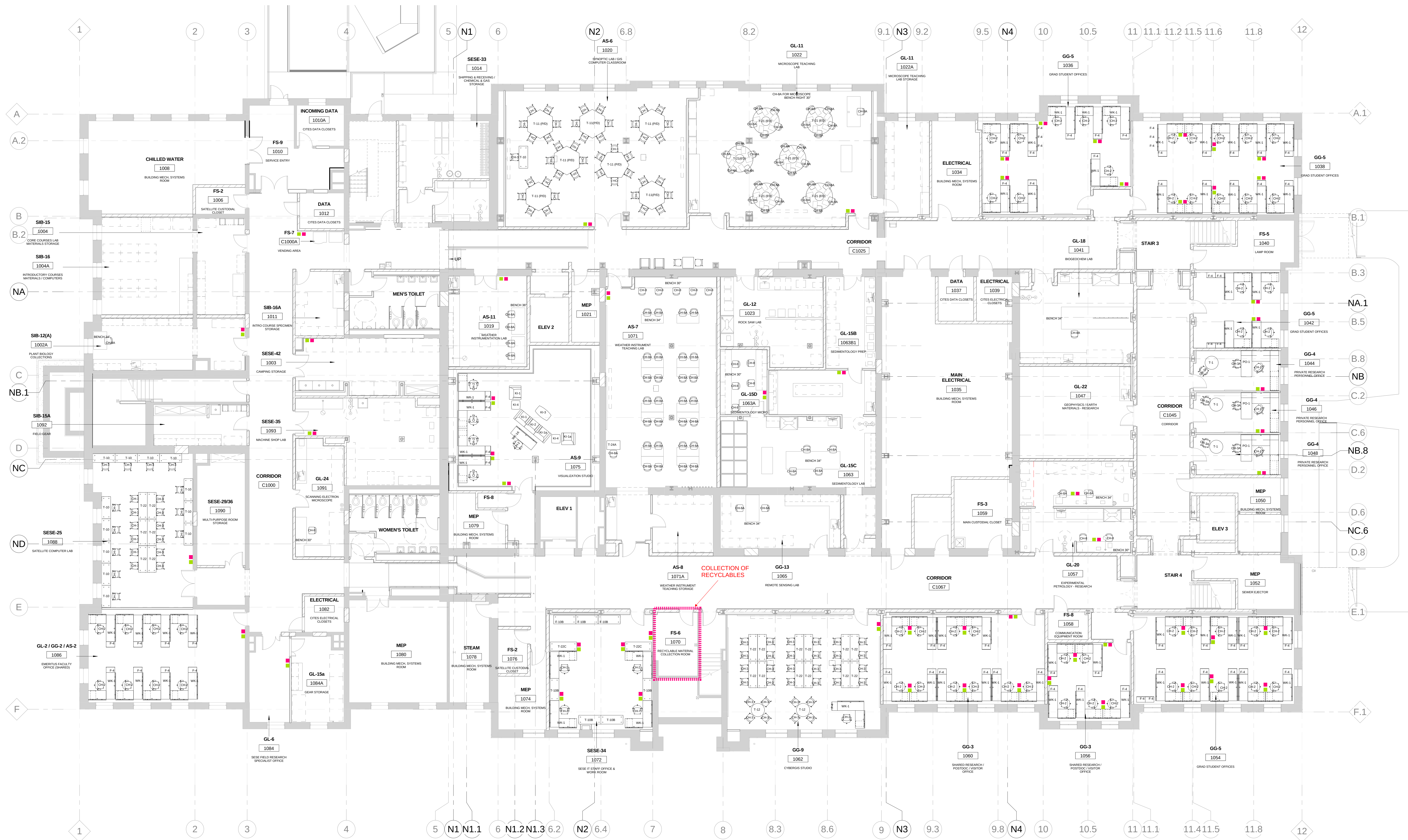
1 LEVEL 1 - FURNITURE SCALE: 1/8" = 1'-0"
